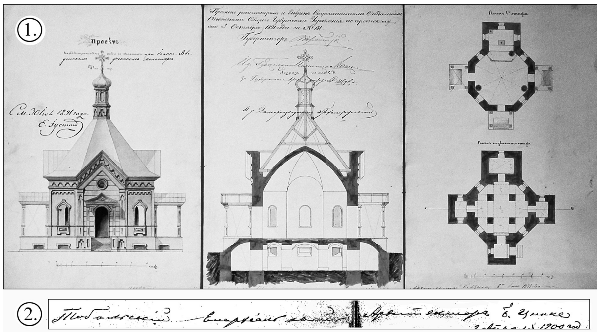
Рис. 2. Материалы из фондов Тобольского историко-архитектурного музея-заповедника (ТИАМЗ). 1 — проект кладбищенской церкви со склепом; 2 — автограф Б. Цинке на плане Иоанно-Введенского монастыря
